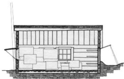
SECTION B-B SCALE: 3/8" = 1'-0"
