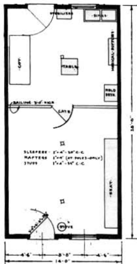
INFIRMARY 14'-0\"/>
